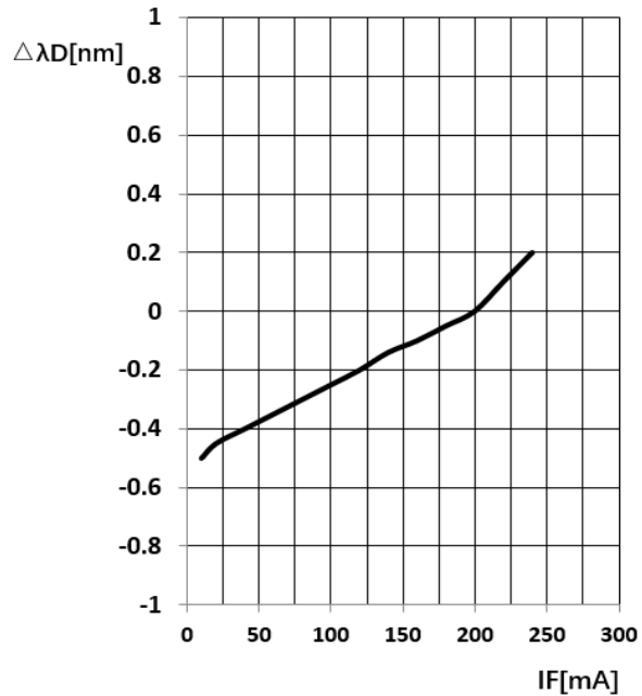
Fig 7. 波长偏移/ Shift in Wavelength
