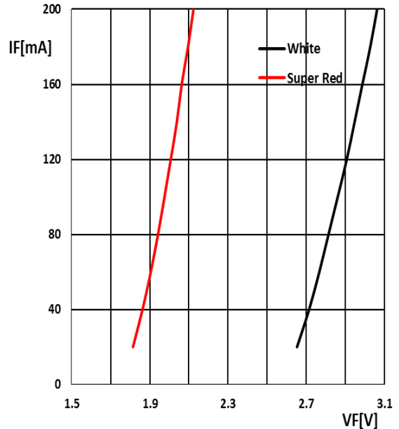
Fig 3. 正向电流 / Forward Voltage
