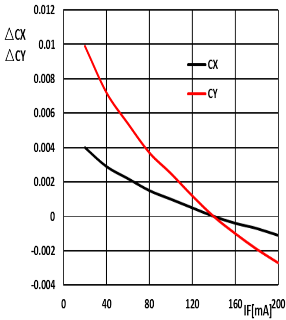
Fig 6. 色坐标偏移/ Chromaticity Coordinate Shift
